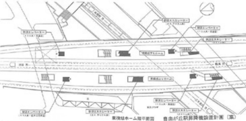
東横線ホーム横断面図 自由が丘駅昇降機設置計画(案)
